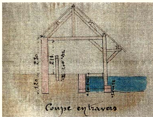
Coupe du lavoir des Bassières, 1891 (AD 28 2 O 307).
